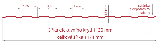
Fasádní profil
