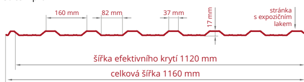
Střešní profil
